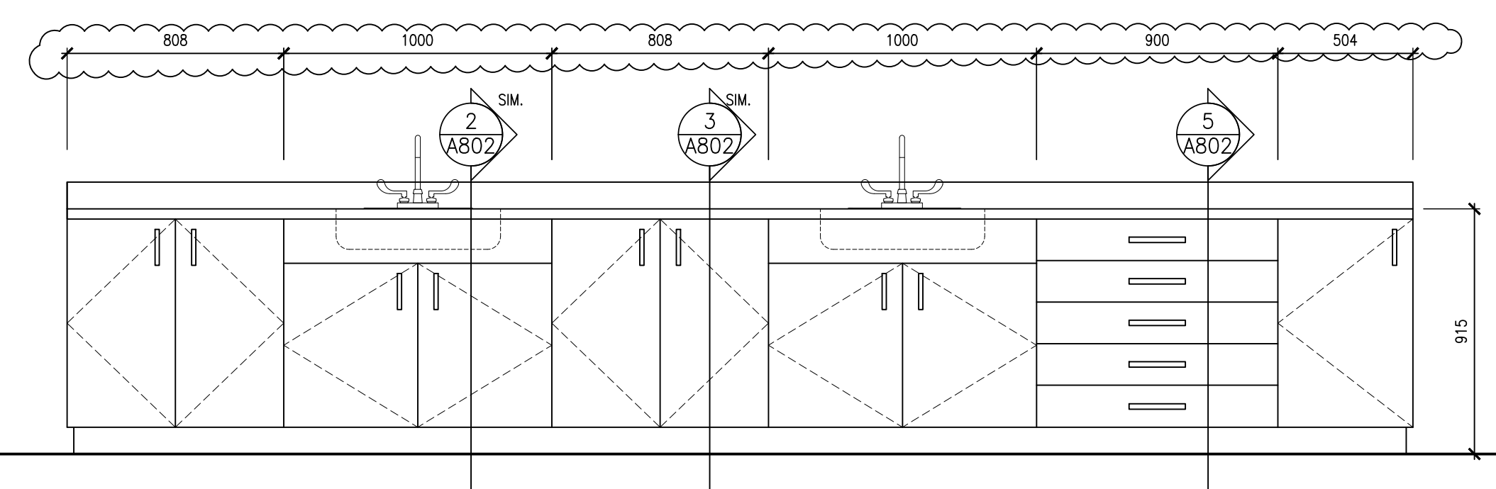
ML-1 ELEVATION
