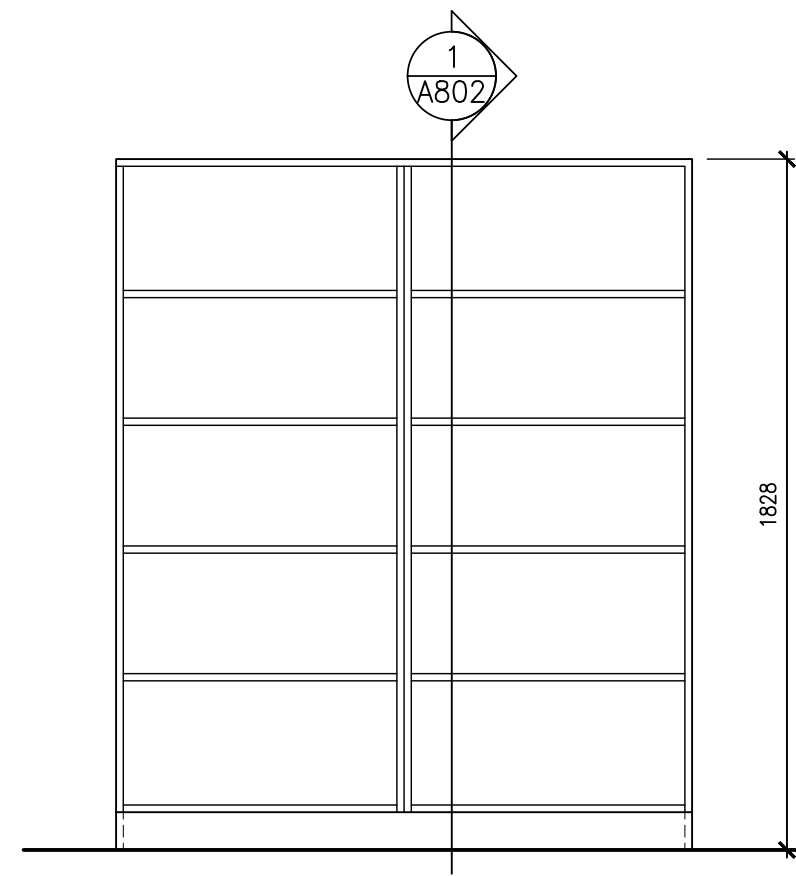
ML-3 ELEVATION
